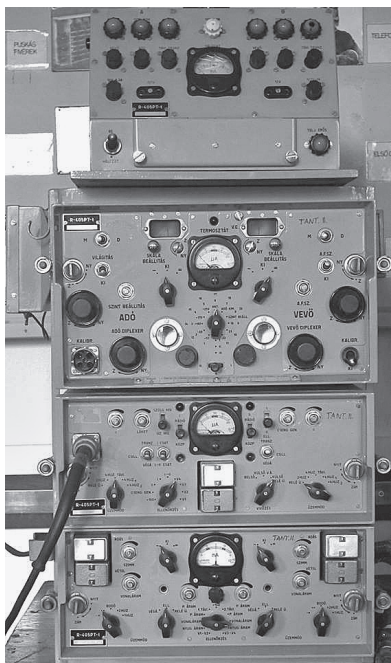
R-405 PT rádiórelé-berendezés
