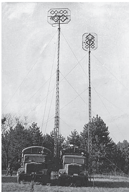
R-1412 rádiórelé-állomás
