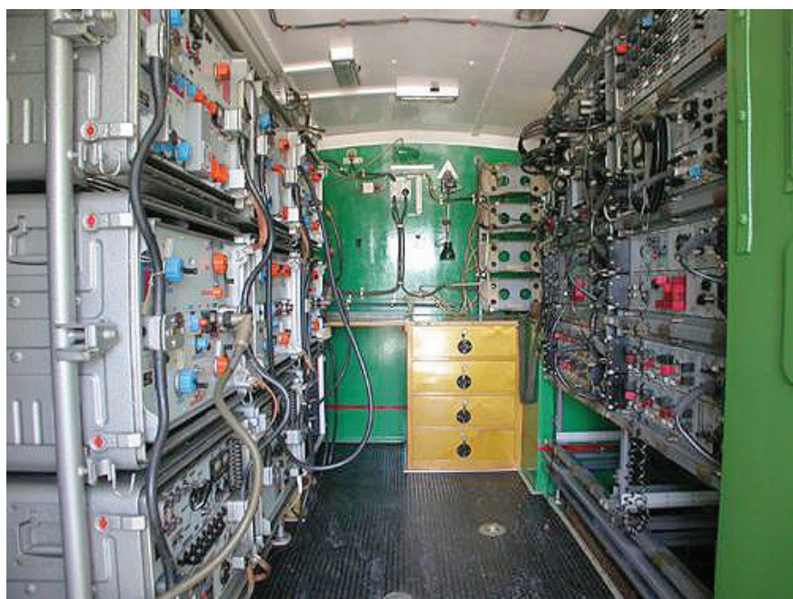
R-1406 rádiórelé-állomás belső tere
