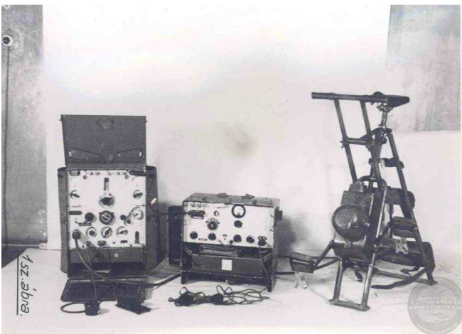
R-7 adó-vevő mobil állomás
