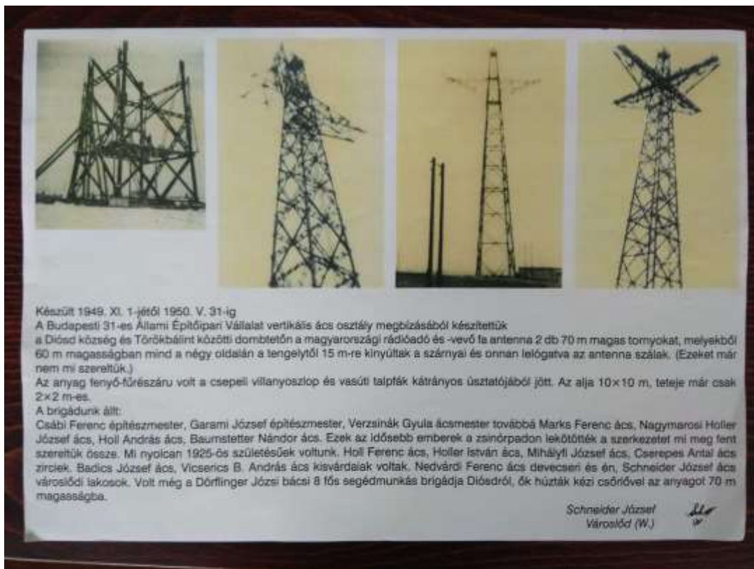
Diósd, Rádió-adóállomás 2db 70m magas antennatorony építése az építésben résztvevő Schneider József képei és visszaemlékezése alapján!
